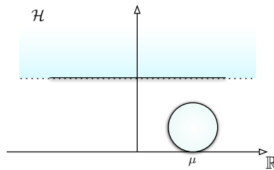
FIGURE 19: Sur la définition de horodisques. Montrés sont deux horodisques, de centre \infty et \mu \in \mathbb{R} .
