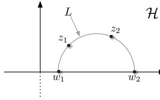
FIGURE 6: Sur théorème 1.5.3.
