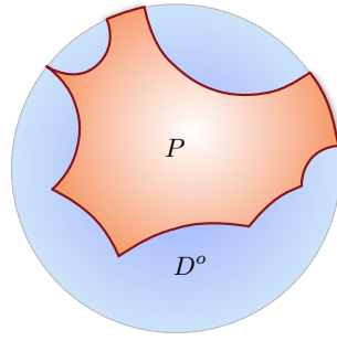
FIGURE 16: Sur théorème 4.2.3 : Exemple d'un polygone généralisé dans le modèle du disque.
