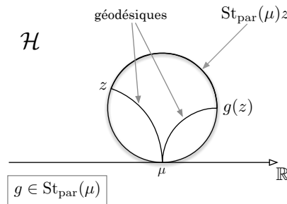
FIGURE 20: Sur lemme 4.3.4 : Les horodisques de centre \mu \in \partial\mathcal{H} sont exactement les orbites de \text{St}_{\text{par}}(\mu) .
