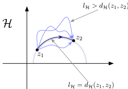
FIGURE 2: Sur la distance des points z_1, z_2 \in \mathcal{H} , réalisée par le demi-cercle droit les contenant.
