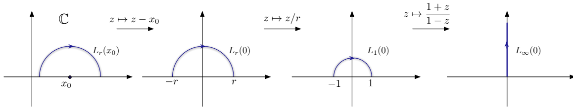
FIGURE 1: Sur la preuve de lemme 1.2.5.
