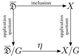
FIGURE 13: Sur théorème 4.1.6. Le diagramme ci-dessus commute.
